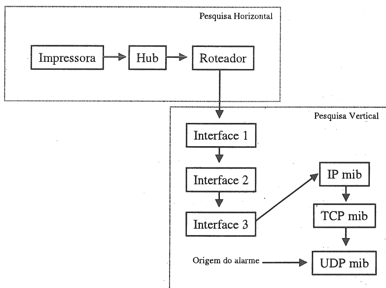
Figura 2 - Algoritmo para identificação de origem de falhas
